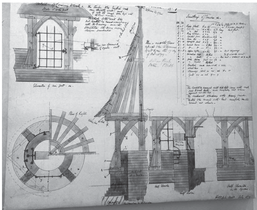
Уэбб Ф. Колодец, калитка сада. Планы, разрезы, фронтальные виды. Около 1861. Галерея Уильяма Морриса. Лондон
