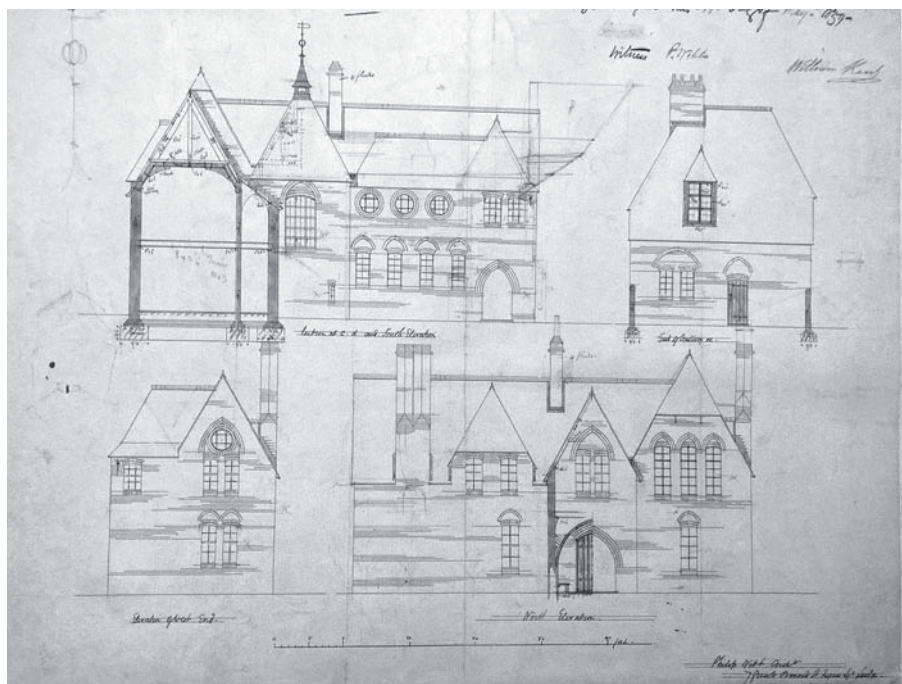
Уэбб Ф. Фасады и разрезы Ред хауса. Около 1861. Галерея Уильяма Морриса. Лондон
