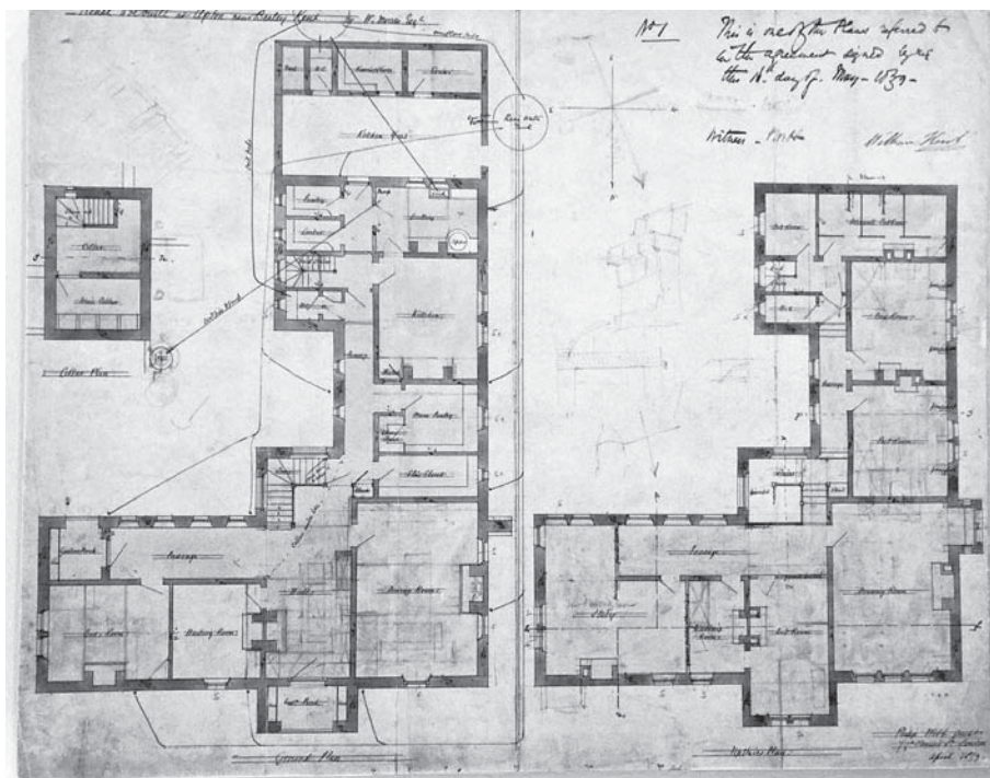
Уэбб Ф. Планы 1-го и 2-го этажей Ред хауса. Около 1861. Кар., сепия, отмывка по бум. Галерея Уильяма Морриса. Лондон
